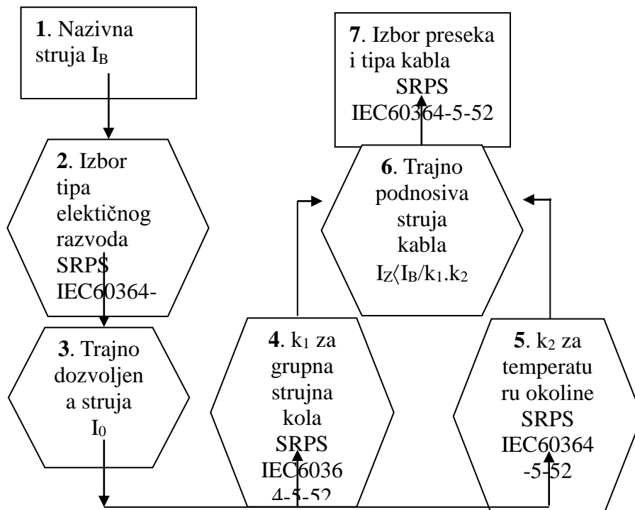
Slika 1. Dijagram faze izbora preseka i tipova kabla
